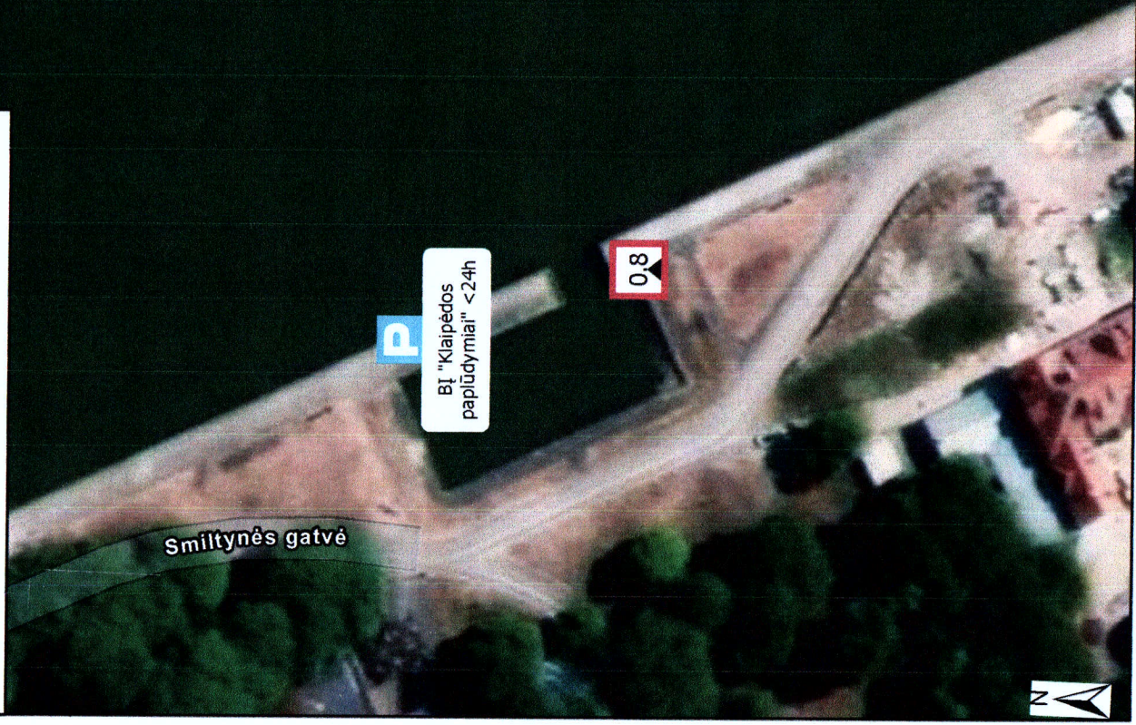
1. Smiltynės krantinės tarp senosios perkėlos ir Smiltynės jachtklubo ženklavimo schema. M 1:1000
